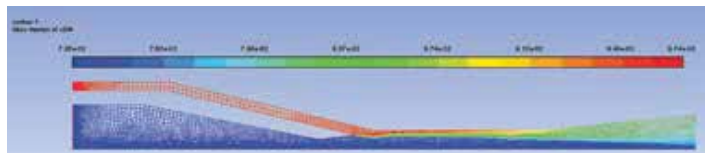
Hình 12. Biên dạng tỷ lệ khối lượng dòng chảy của khí ethane trong hỗn hợp
