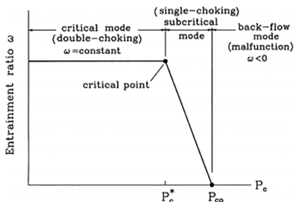
Hình 14. Đồ thị tỷ số hút entrainment so với áp suất ngược [24]
