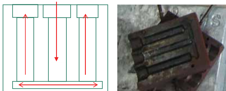
Hình 3. Bộ khuôn đúc mẫu thử nghiệm
